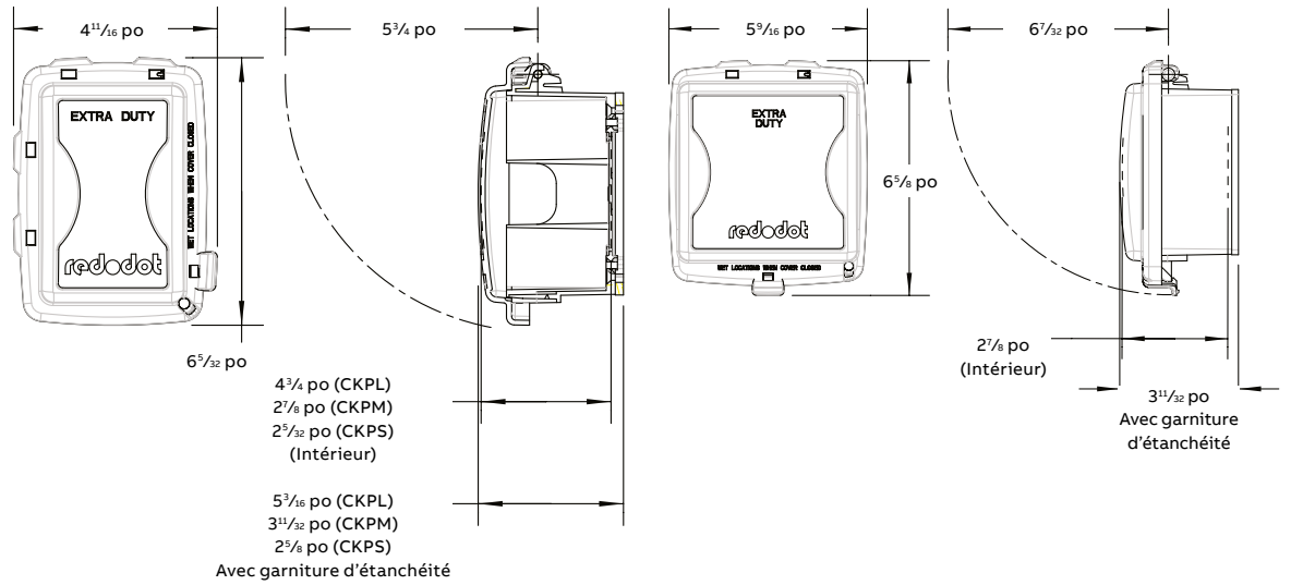
Un groupe (CKPM) – dimensions
