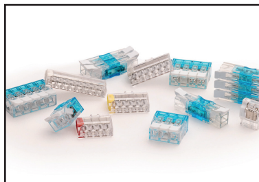
Marrette MD Série PRO-Snap Connecteurs de fils
