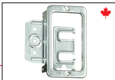
Iberville Supports pour câbles basse tension
